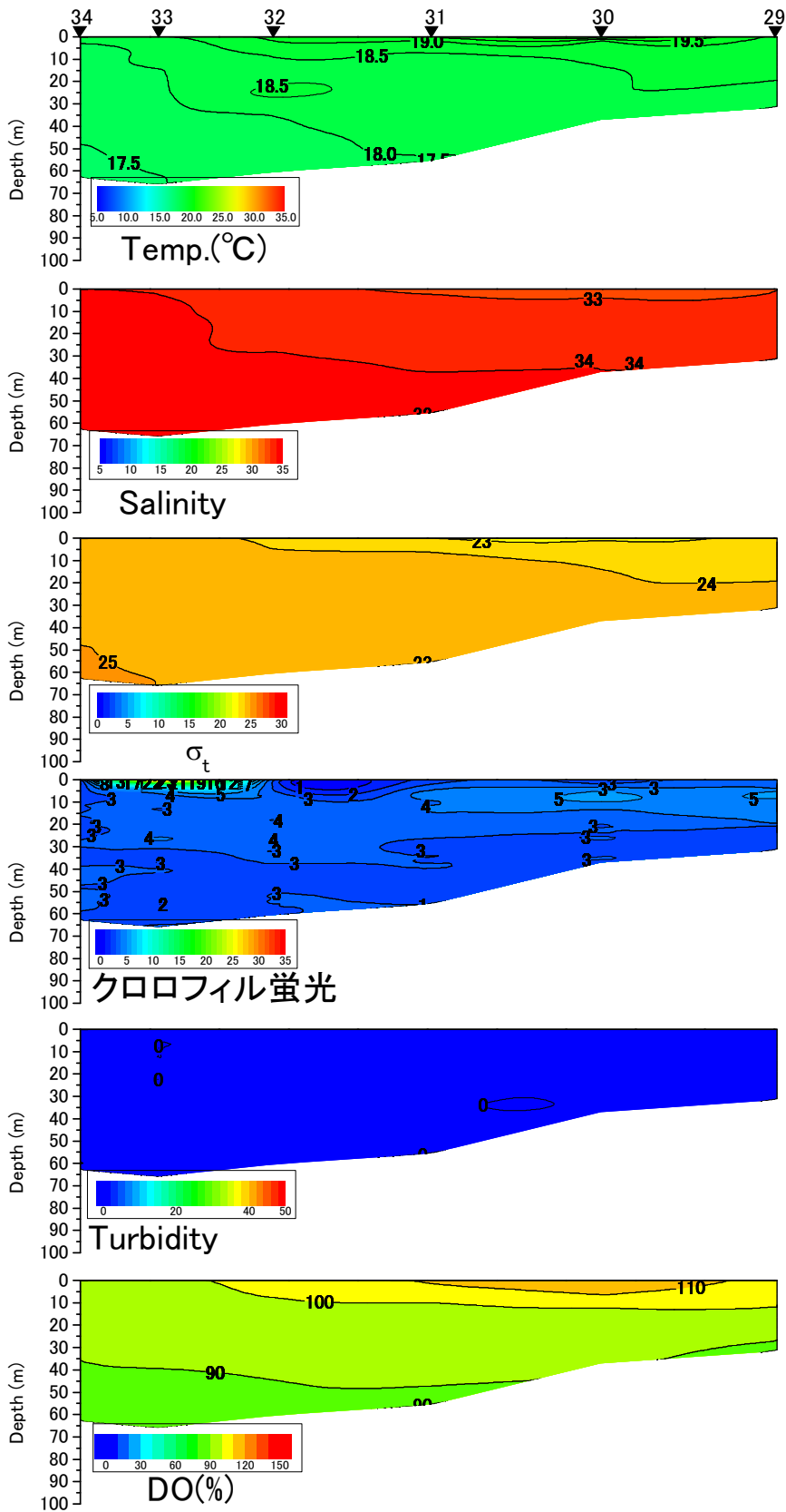
八代海西ラインの水温(°C)、塩分、密度( \sigma_t )、クロロフィル蛍光強度、濁度、溶存酸素飽和度(DO%)の鉛直面図(国土交通省の調査による) (2017年5月17日)
